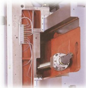
Y-Achsen-Stufenkonstruktion( SD+SV)
